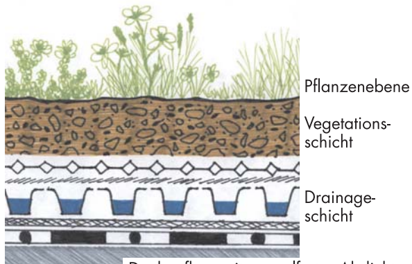
Dachaufbau mit wurzelfester Abdichtung
